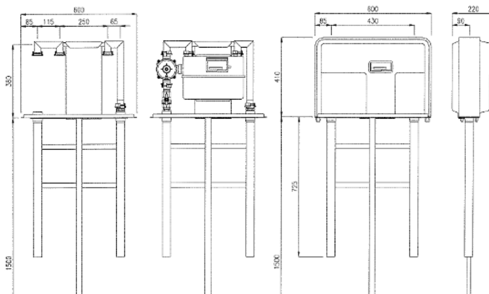
M2/2-9. ábra BORSFÉM gyártmányok kisnyomású (legfeljebb 33 mbar), és középnyomású fogyasztói vezetékhez
