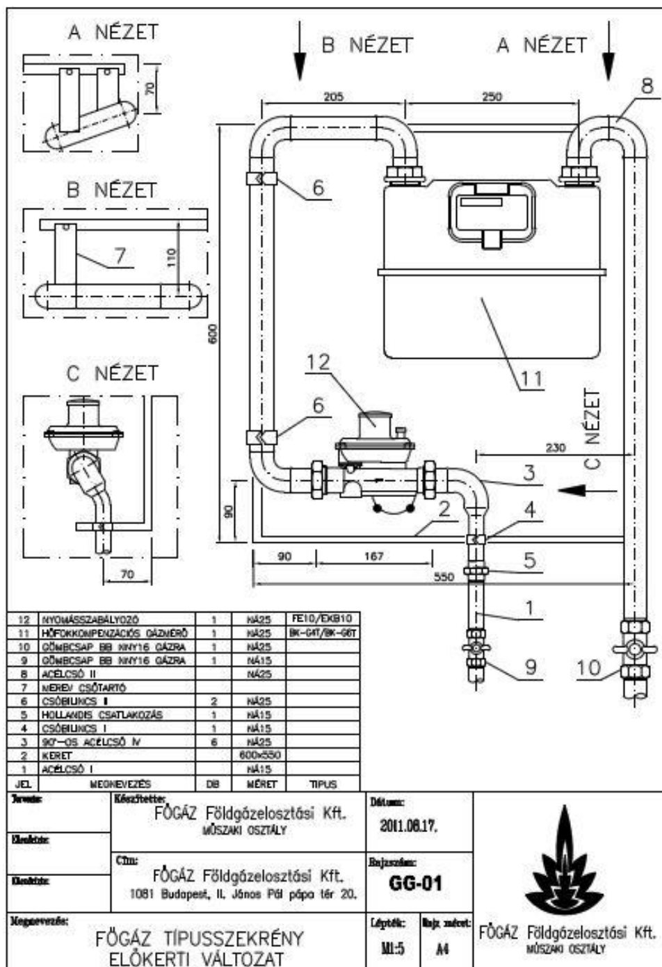
M2/2-1 ábra: FŐGÁZ típus szekrény, előkerti változat
