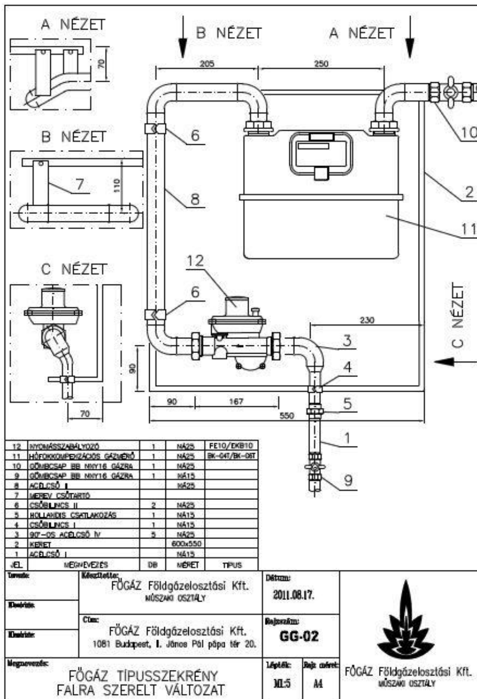
M2/2-2 ábra: FÖGÁZ típusszekrény, falra szerelt változat
