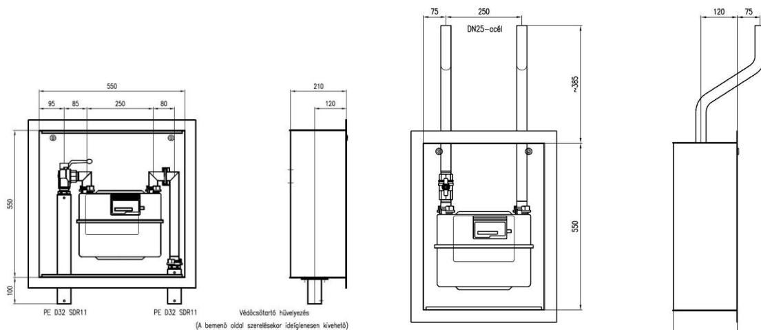
M2/2-3. ábra: Kisnyomású mérőkötés előkerti, fali és süllyesztett megoldásokhoz, fogyasztói vezeték kivezetés lehet: alsó-felső, hátsó
